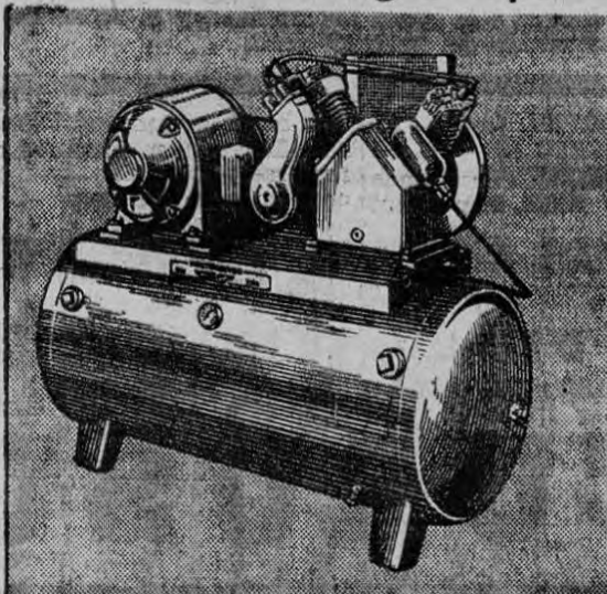
Compresor Worthington Enfrido por Aire, para Tanques, de Dos Etapas, Actuado por Corriente. Los hay de todo tamaño y para todo tipo de transmisión.
